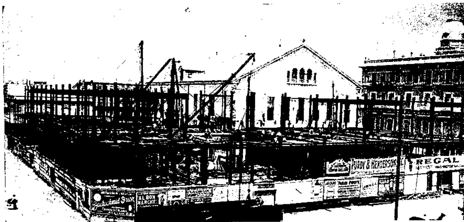
Vista de la armazón de acero, fabricada en los talleres de esta Compañía, del edificio del Centro Gallego, en sus comienzos.
